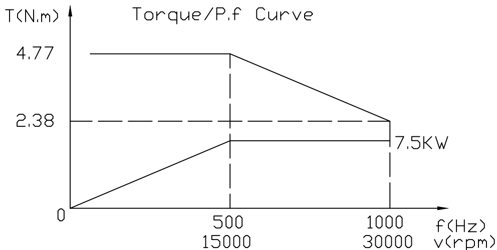
扭矩/功率曲线 Torque/P.f Curve
